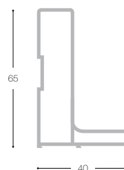
Perfil suplementario vertical lateral
