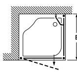
Instalación de 1 Puerta lateral (PL) y de 1 Lateral fijo (LF)
