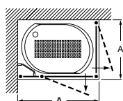
Instalación de 2 Puertas laterales (PLF y PL)
